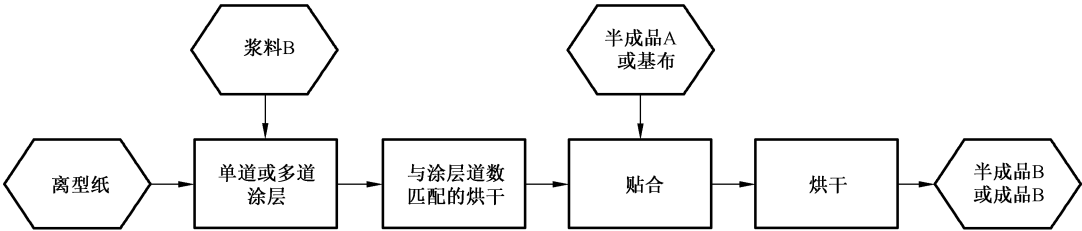
图 2 干法工艺流程示意图
