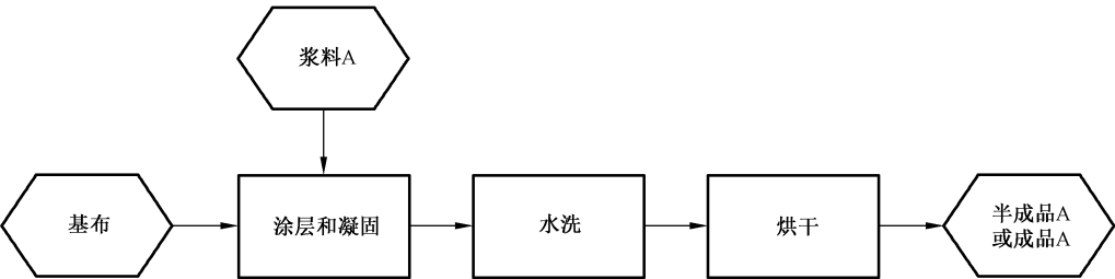
图 1 湿法工艺流程示意图
