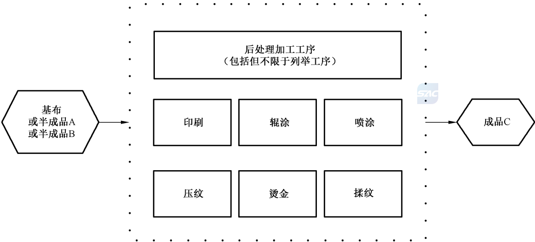
图 3 后处理工艺流程示意图
